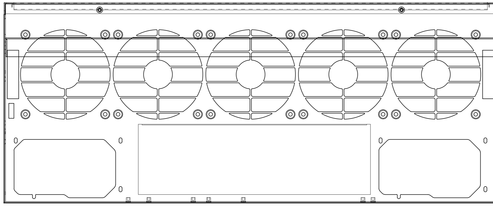
SECTION A-A
